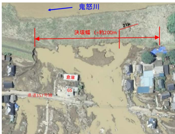
決壊区間航空写真(H27/9/12撮影)
