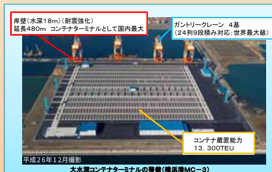
大水深コンテナターミナルの整備(横浜港MC-3)
