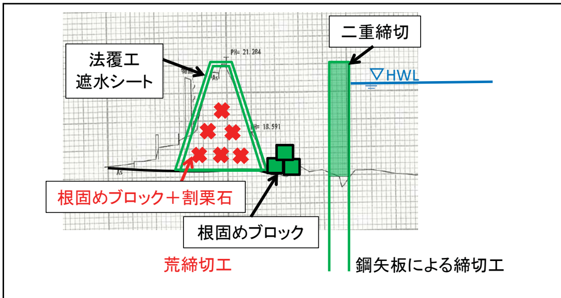
作業ヤードの造成
