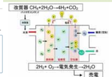
栃木県鬼怒川流域下水道県央浄化センターにおける消化ガス発電のしくみ
