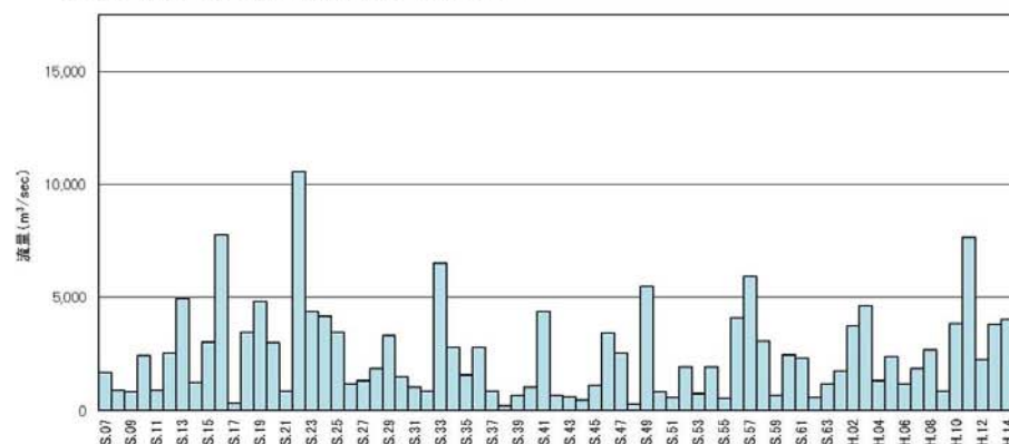
年最大流量(岩淵地点)の経年変化
