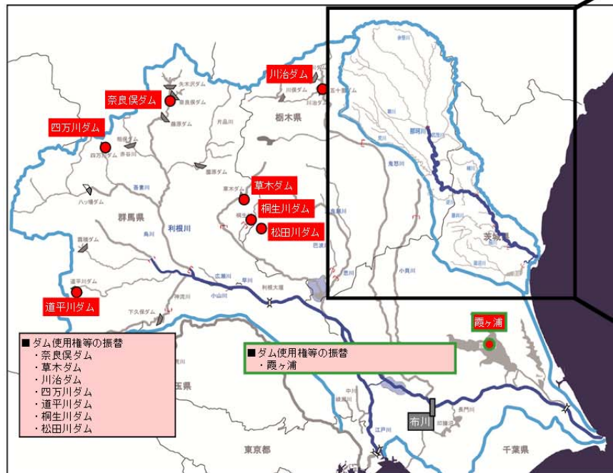
図 4.3-65 新規利水対策案の概要 ケース 4 ダム使用権等の振替による新規利水対策案
