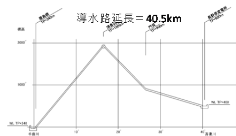
図 4.3-29 導水路縦断面図
