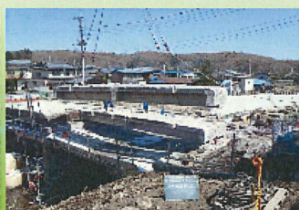
コンクリート桁切断撤去中
