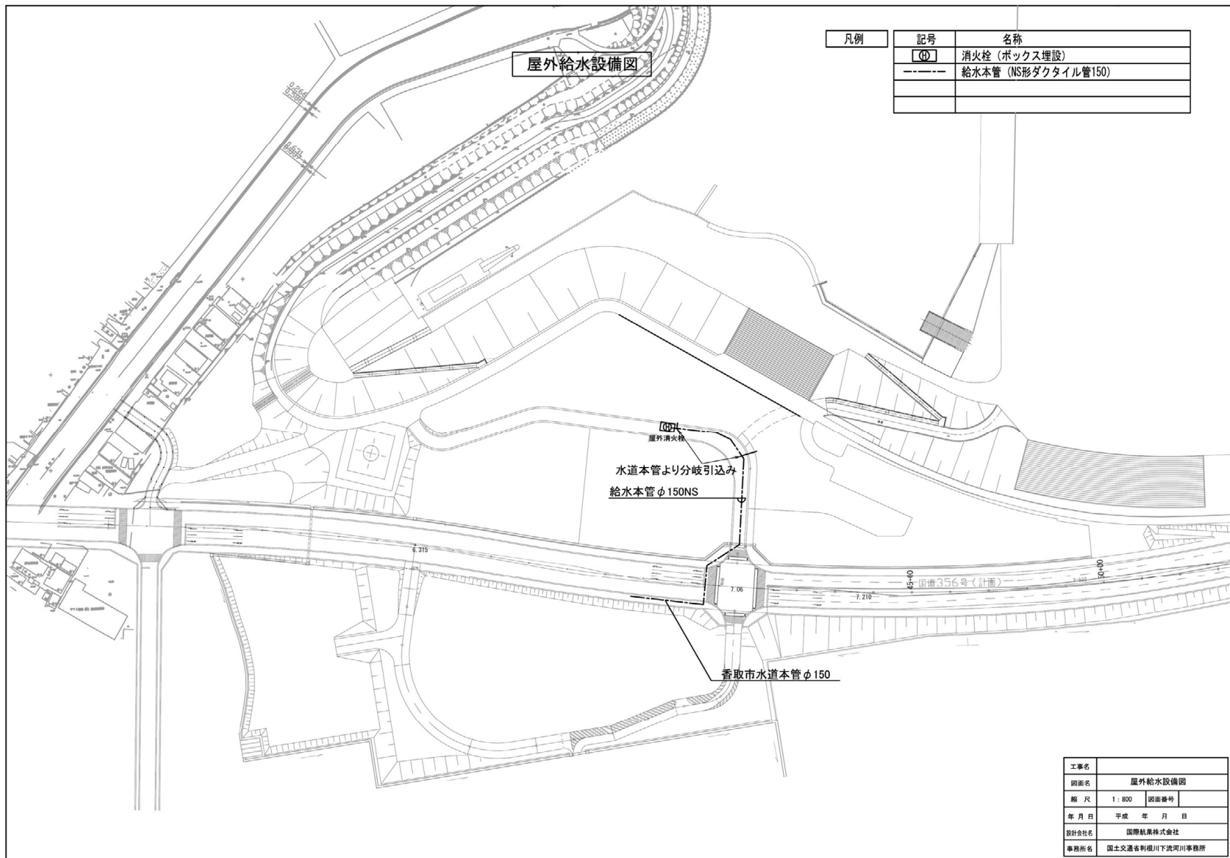
参考図-10 (1) 供給処理施設引き込み図 (給水設備計画図)
