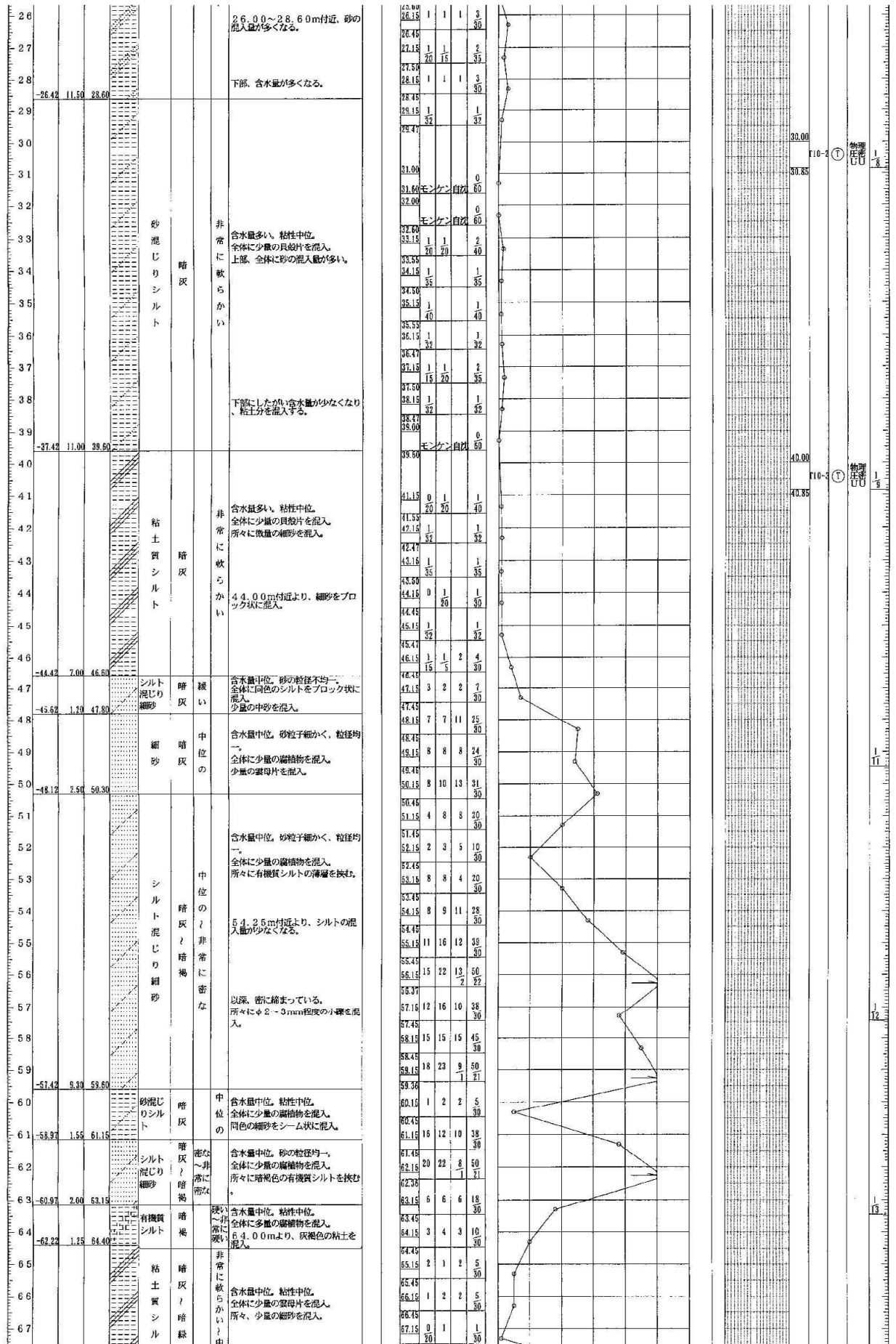
参考図-8(12) ボーリング柱状図(本宿-10)
