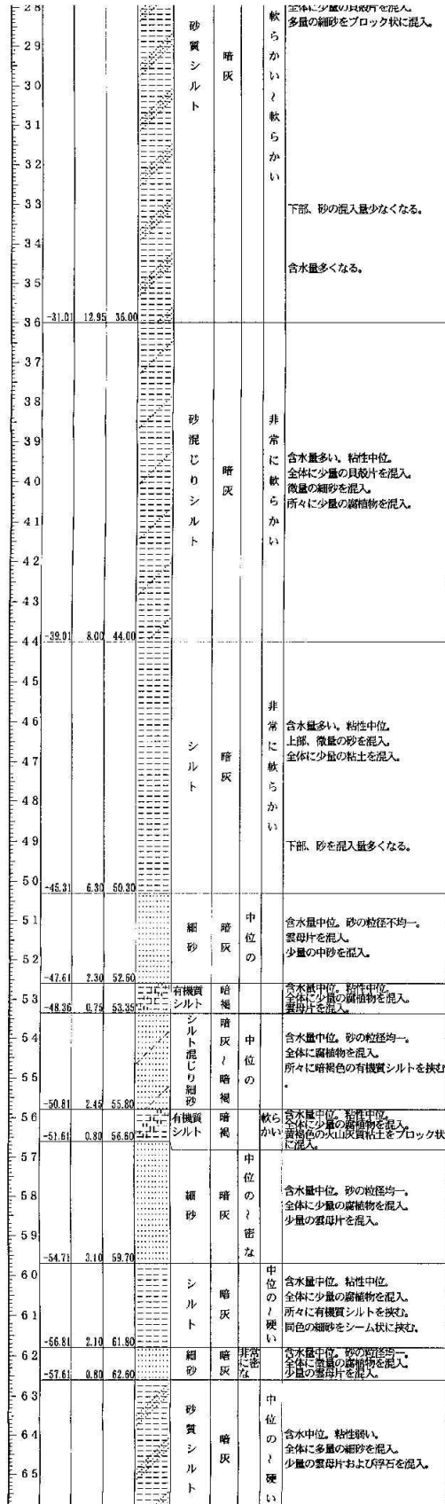
参考図-8(9) ボーリング柱状図(本宿-8)
