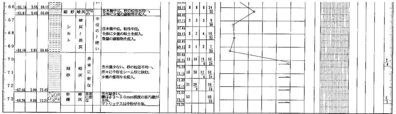
参考図-8(10) ボーリング柱状図(本宿-8)
