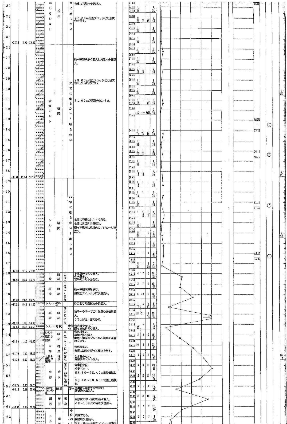
参考図-8(6) ボーリング柱状図(No. 1)
