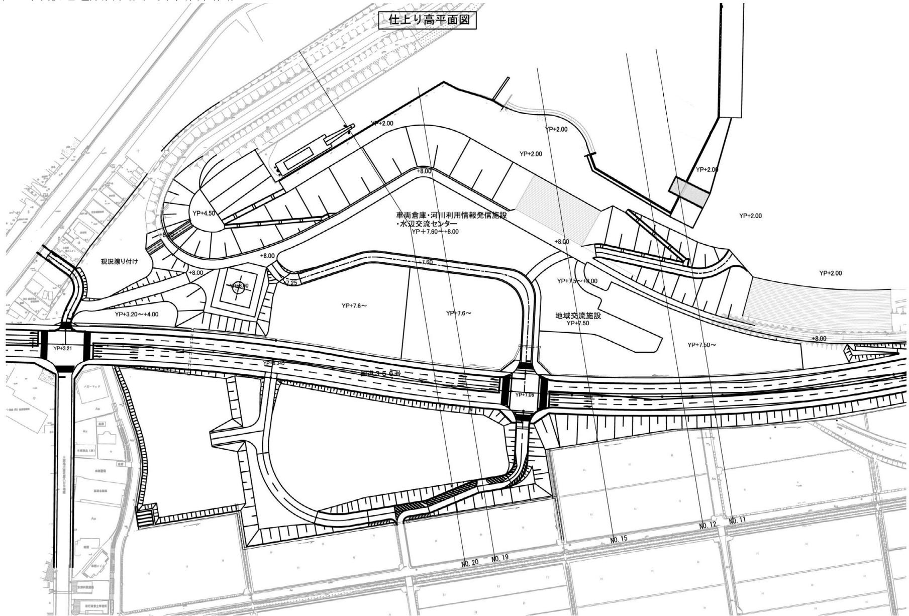
参考図-7 (1)敷地造成計画図 (平面計画図)
