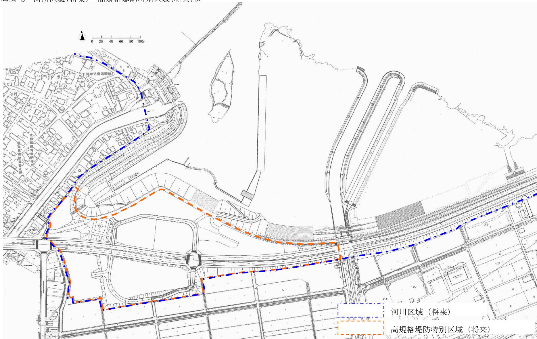
参考图-3 河川区域(将来)・高規格堤防特別区域(将来)図
