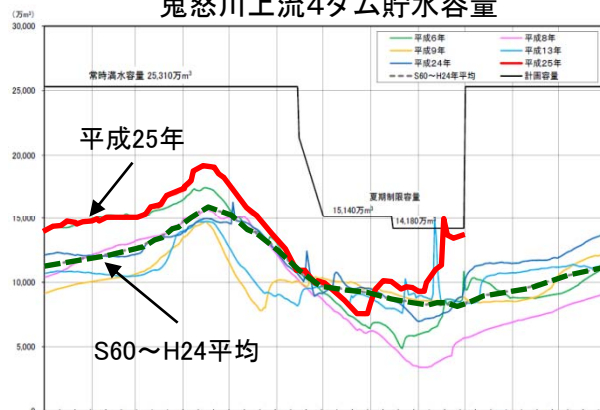
鬼怒川上流4ダム貯水容量
