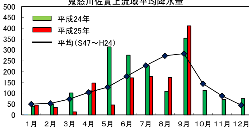
鬼怒川佐貫上流域平均降水量
