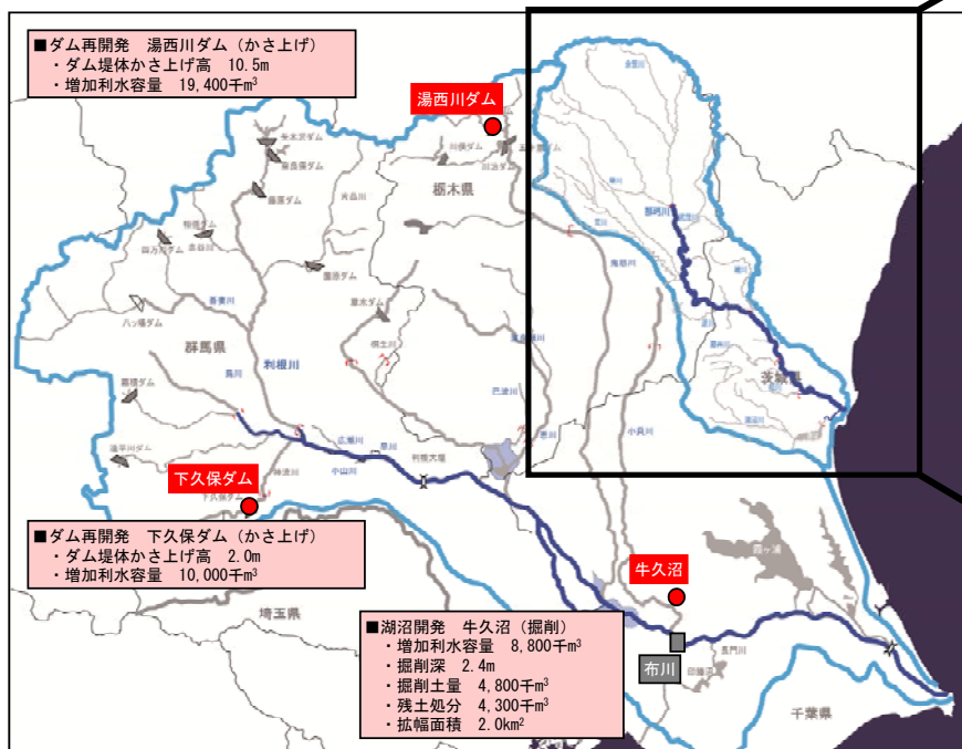
図 4.3-62 新規利水対策案の概要 ケース 1-2 利根川で 4.826m 3 /s の開発量を確保し、霞ヶ浦に導水する新規利水対策案
