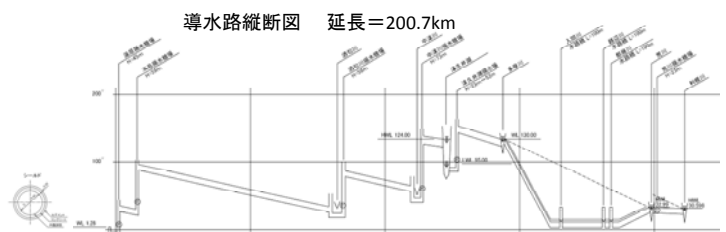
図 4.3-27 導水路縦断面図
