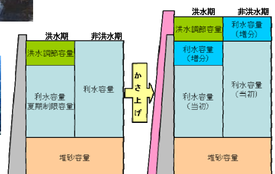
図 4.3-21 かさ上げイメージ図
