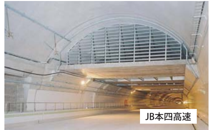
電気集じん機室の例
