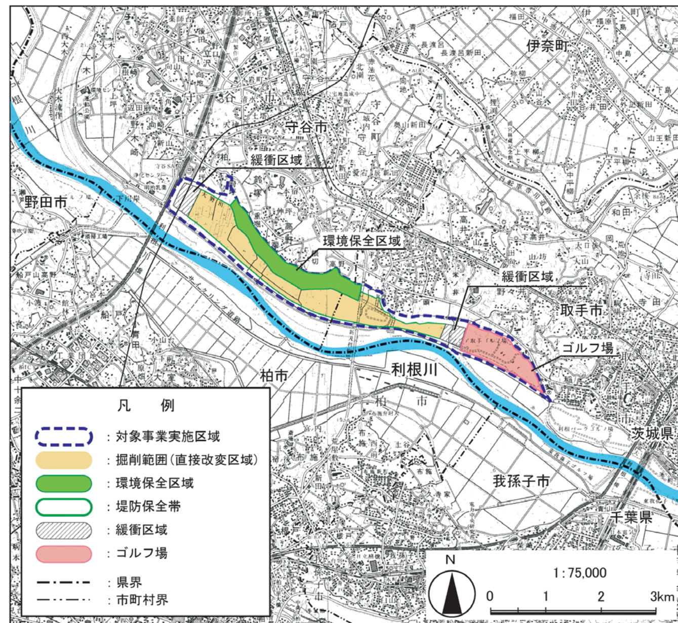
図 1 稲戸井調節池掘削事業計画 概要図
