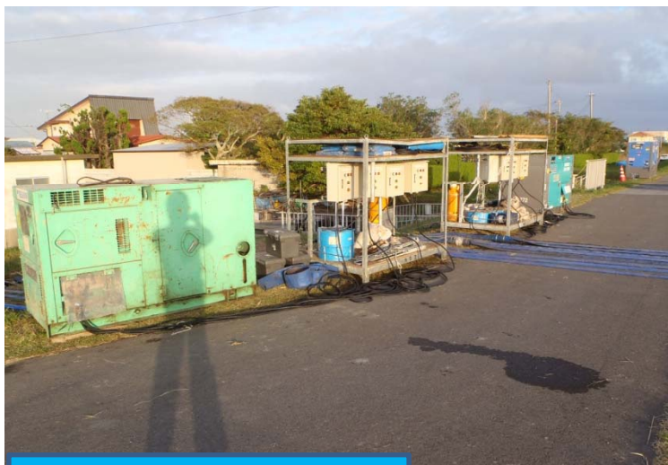
排水ポンプ設置状況(10月25日)
