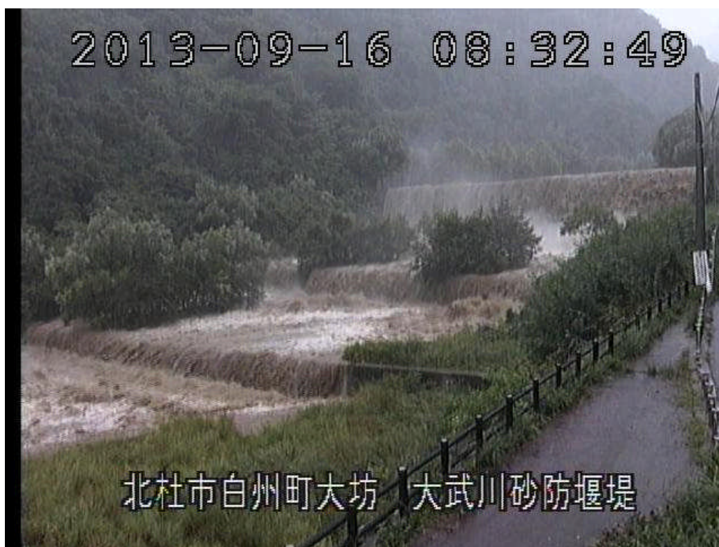
大武川砂防堰堤 出水状況（9月16日8時頃撮影）
