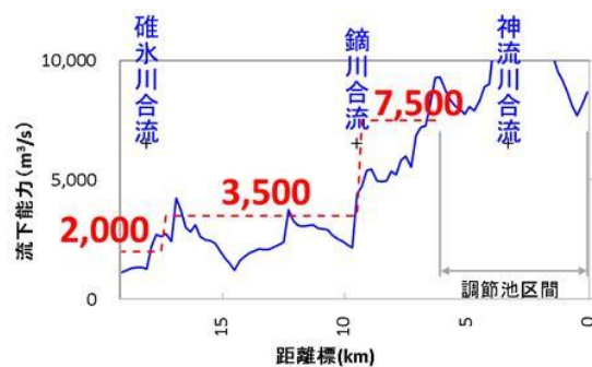
図 4-3 利根川の河道目標流量
