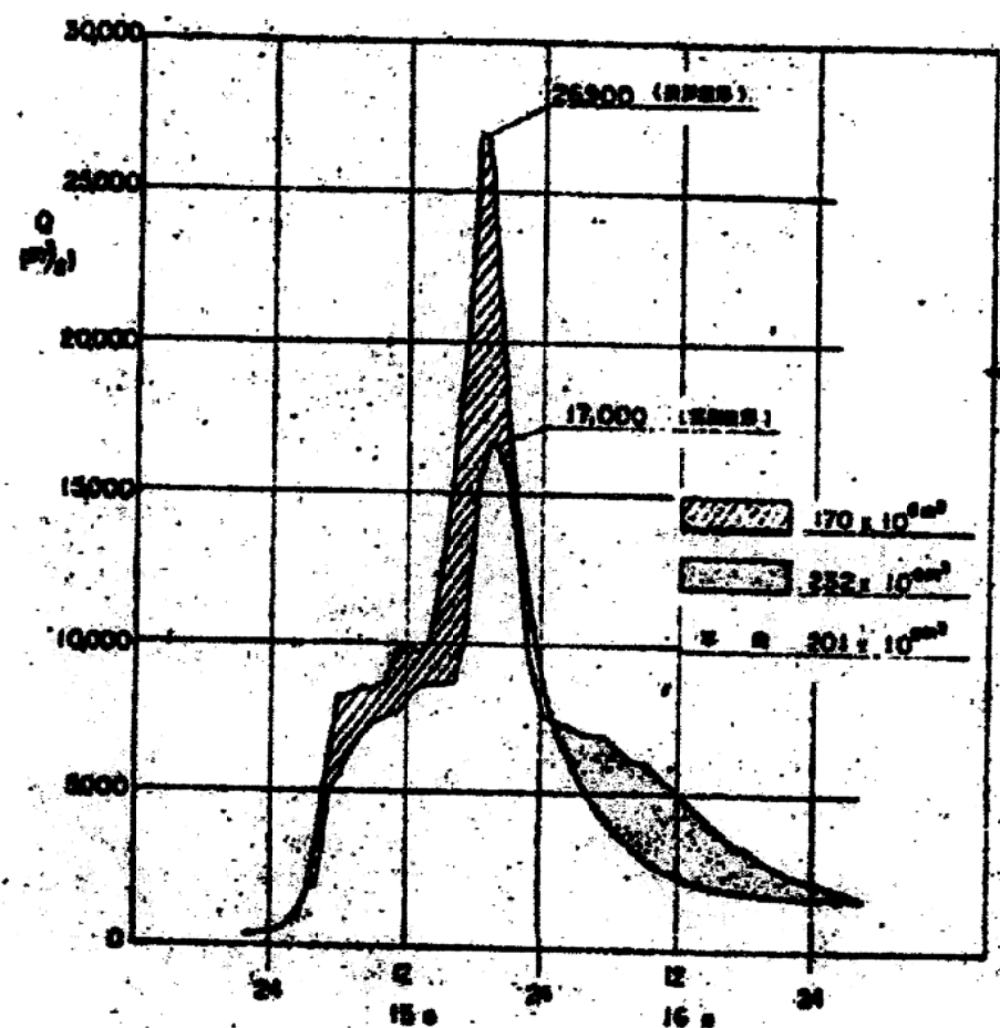
図8 昭和45年ごろ推算されていたカスリーン台風最大流量26900 m³/秒と実績流量17000 m³/秒の差である八斗島上流での氾濫量約2億m³の説明図 (出典:「利根川上流域における昭和22年9月洪水(カスリーン台風)の実態と解析」(利根川ダム統合管理事務所、昭和45年4月))
