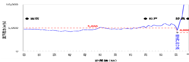
図 4-2 江戸川の河道目標流量
