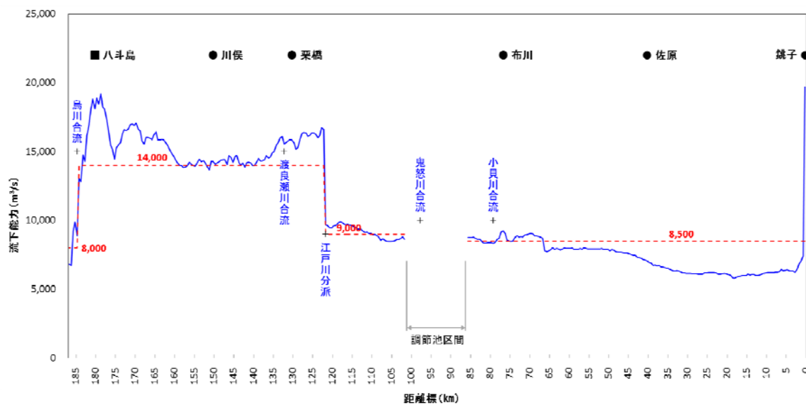
図 4-1 利根川の河道目標流量
