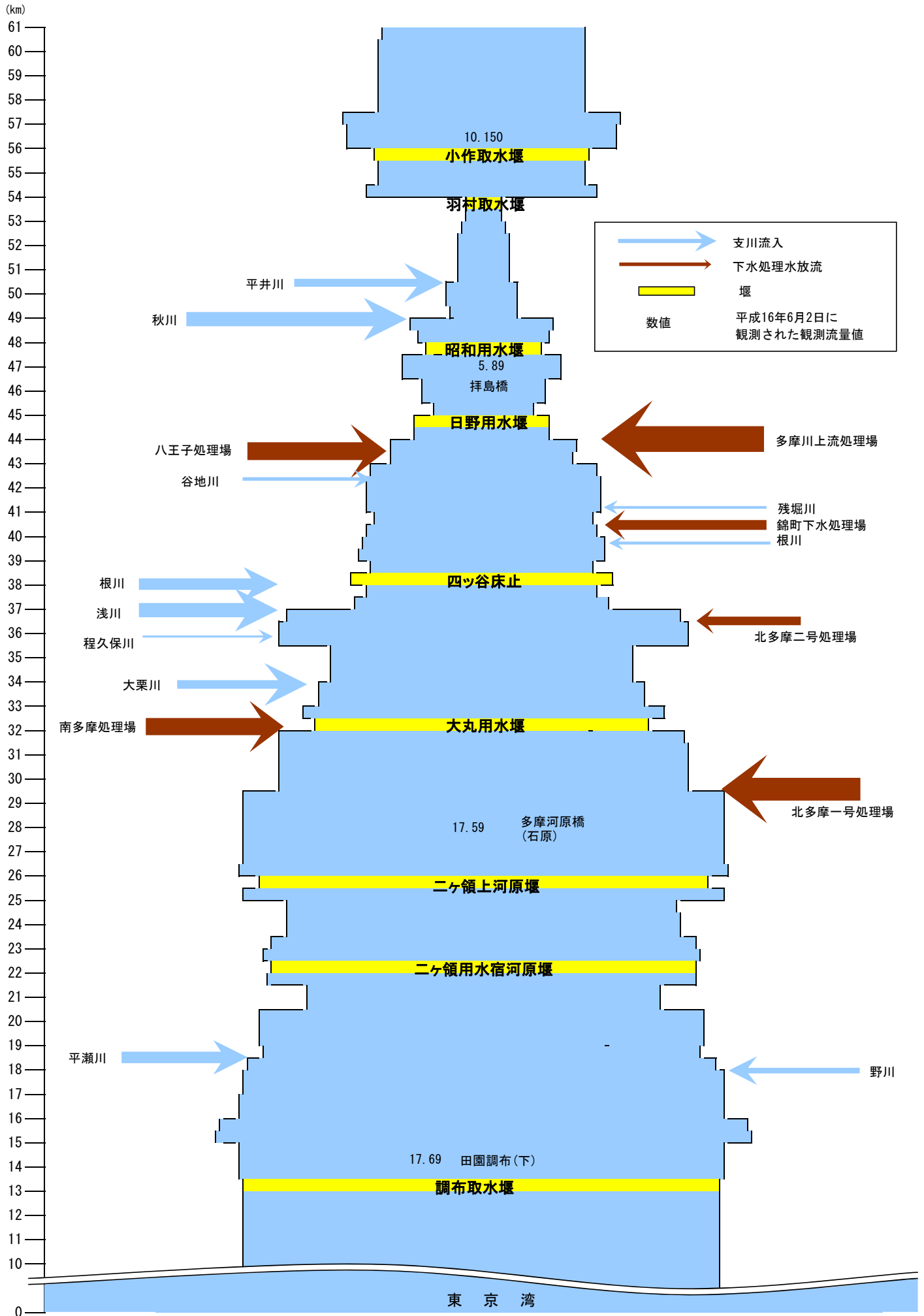
多摩川流況模式図(灌漑期)
