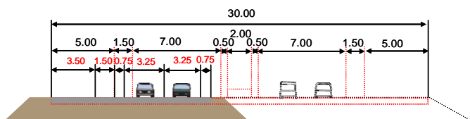
断面図
