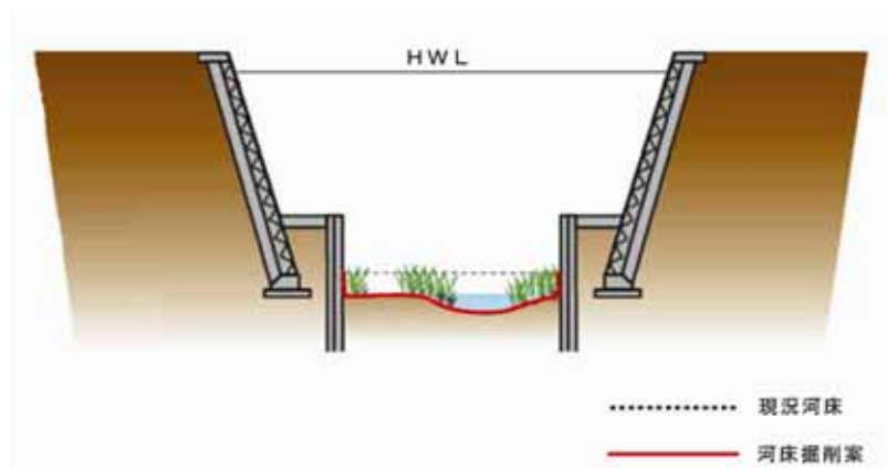
図 4.24 八反下橋付近代表断面
