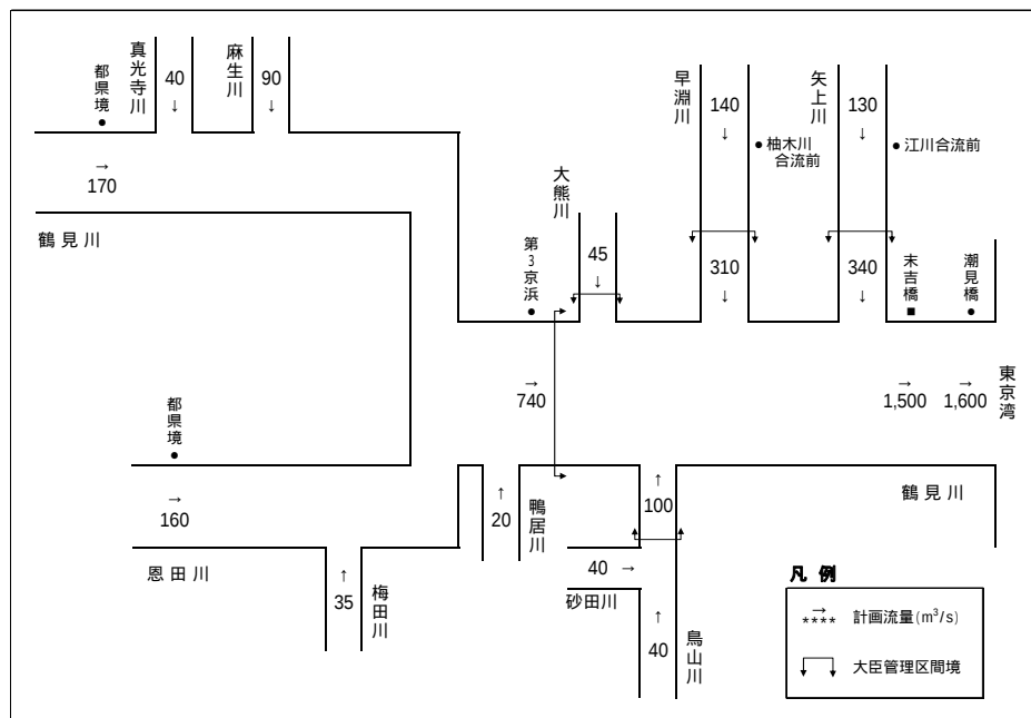
図 3.2 鶴見川整備目標流量
