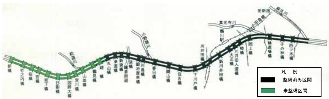
図 4.16 鶴見川（東京都管理区間）整備
