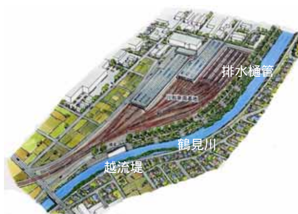
図 4.19 川和遊水地
