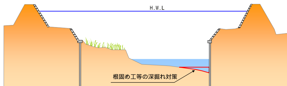
図 4.7 深掘れ対策のイメージ
