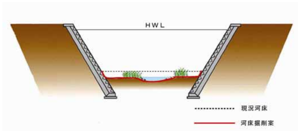
図 4.25 真部橋付近代表断面
