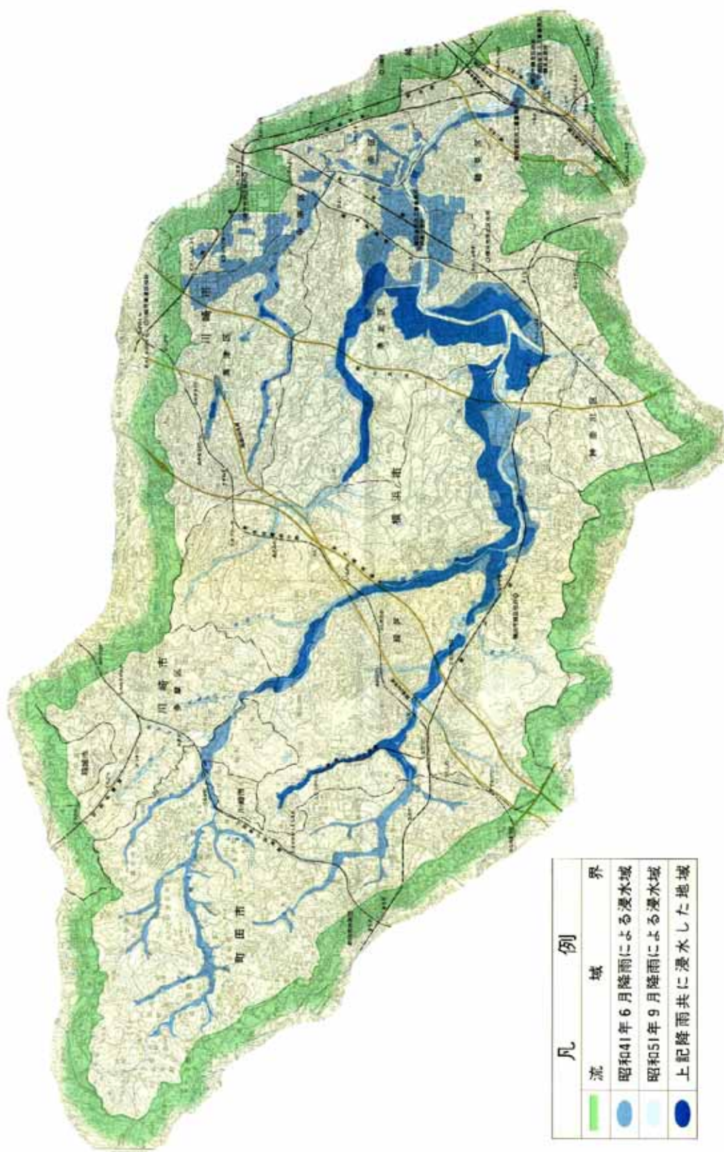
図 2.1 浸水実績図
