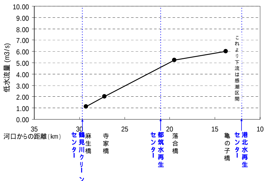
図 2.4 鶴見川本川流量縦断図（平成 15 年）
