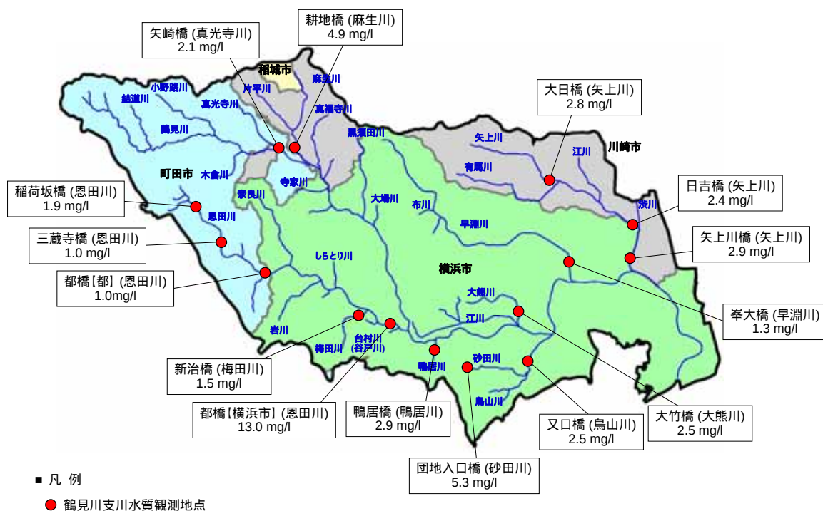
図 2.10 支川における水質測定地点と BOD75%値 (平成 15 年)
