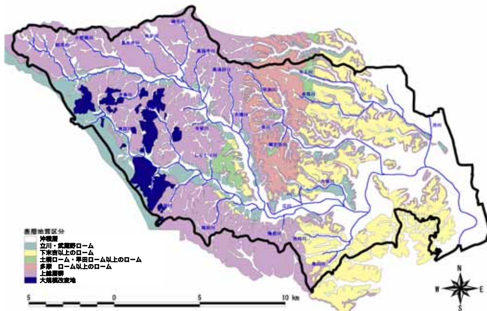
図 1.3 地質図
