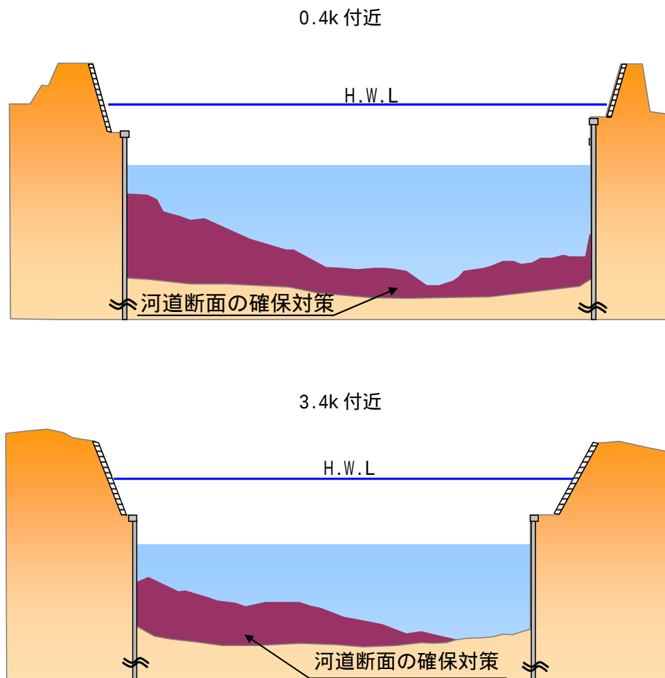
図 4.4 河道掘削断面図
