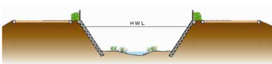
図 4.26 三保天神橋付近代表断面
