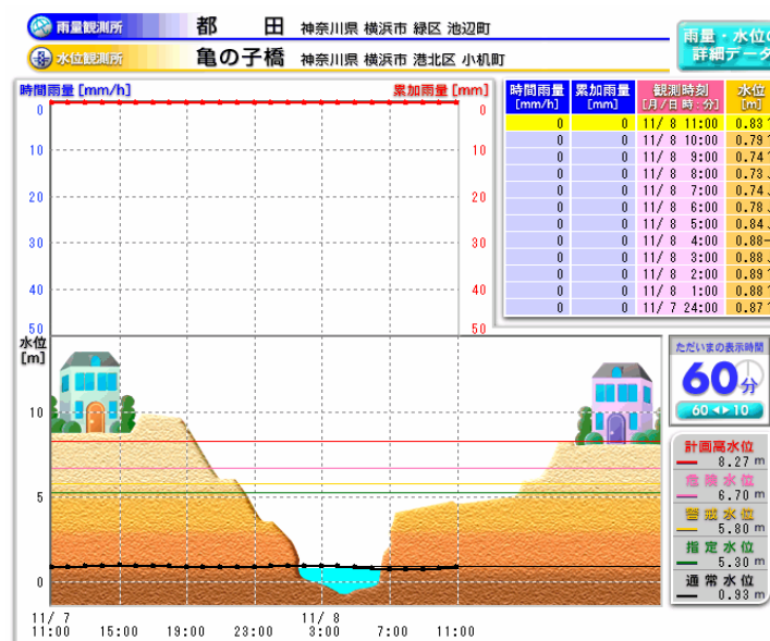
河川横断と水位・雨量の配信状況図 (H16.11.08)
