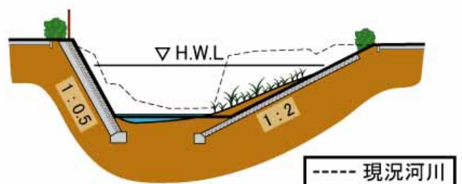
図 4.13 坂下橋付近代表断面
