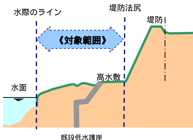
図 4.1 ゾーンの横断方向の対象範囲
