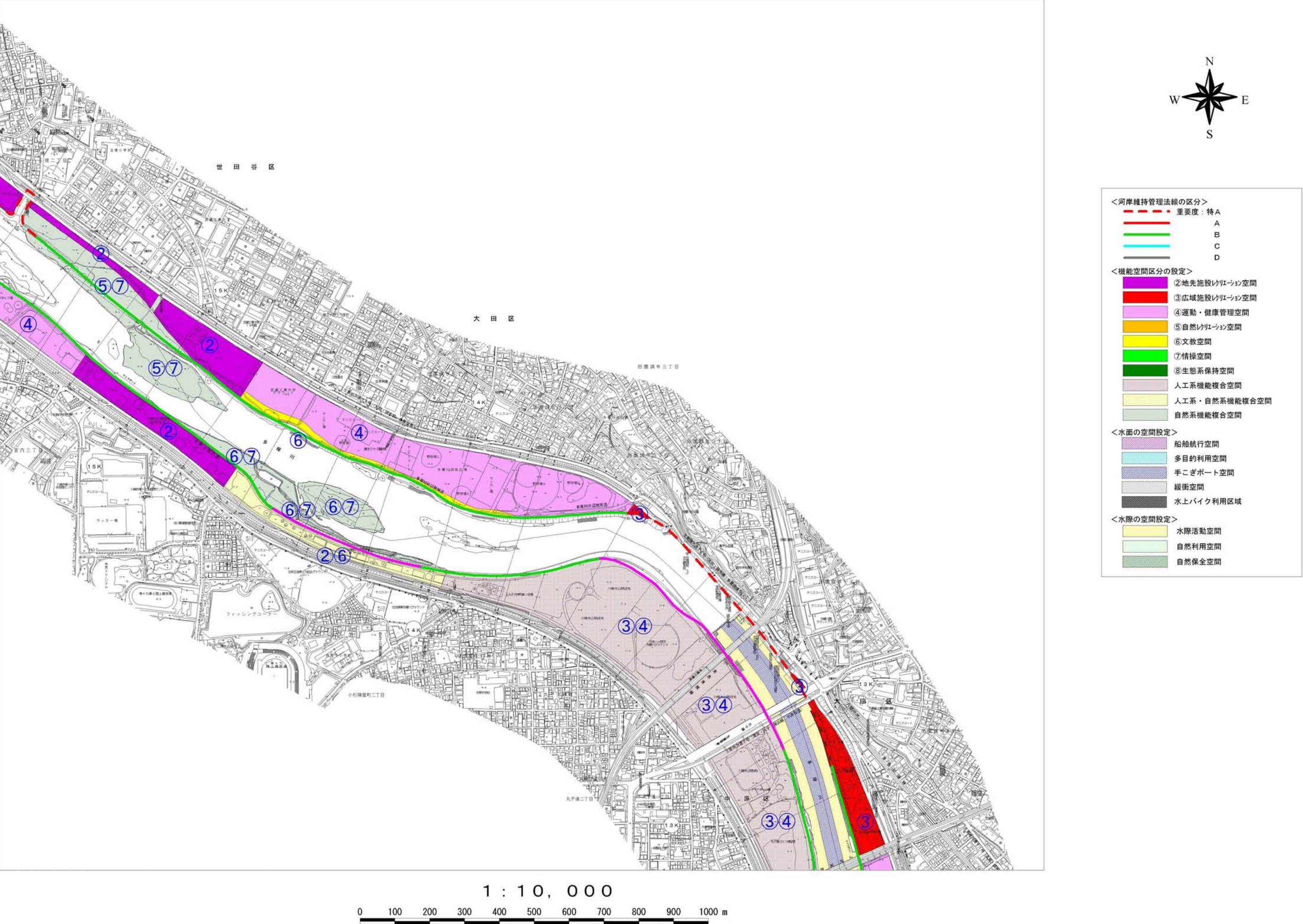
附図（機能空間区分等設定図） 多摩川 No. 07
