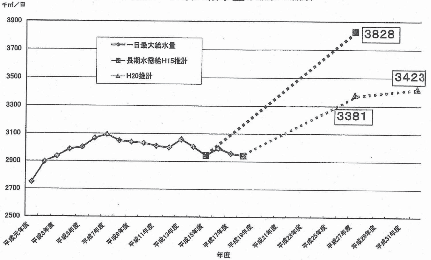
図① 千葉県一日最大給水量(水道用水+工業用水)
