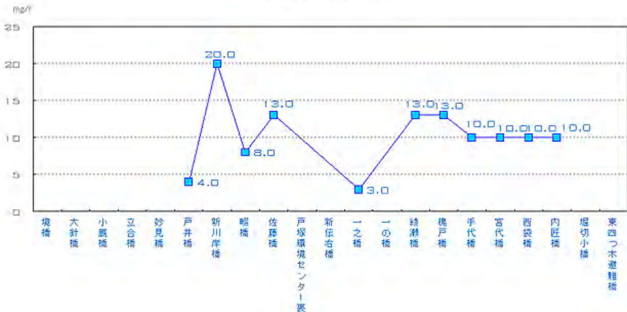
OOD縦断変化図(本川:平成16年度)
