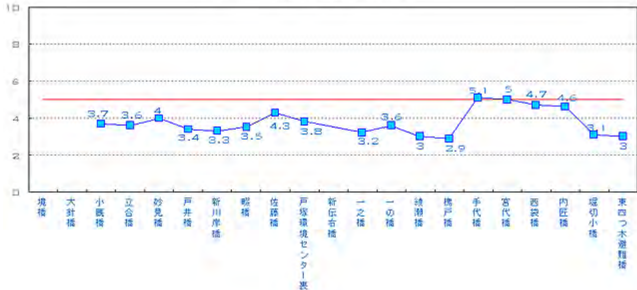
BOD縦断変化図(本川; 平成13年度)
