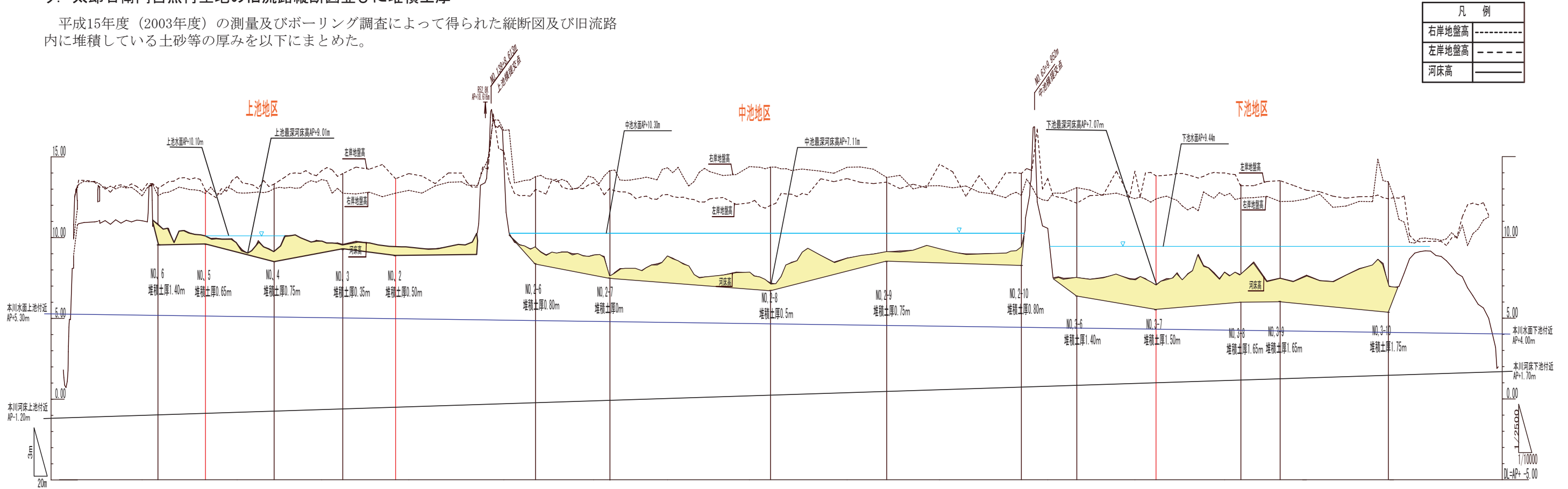
図1-10 旧流路縦断面図（堆積土厚）
