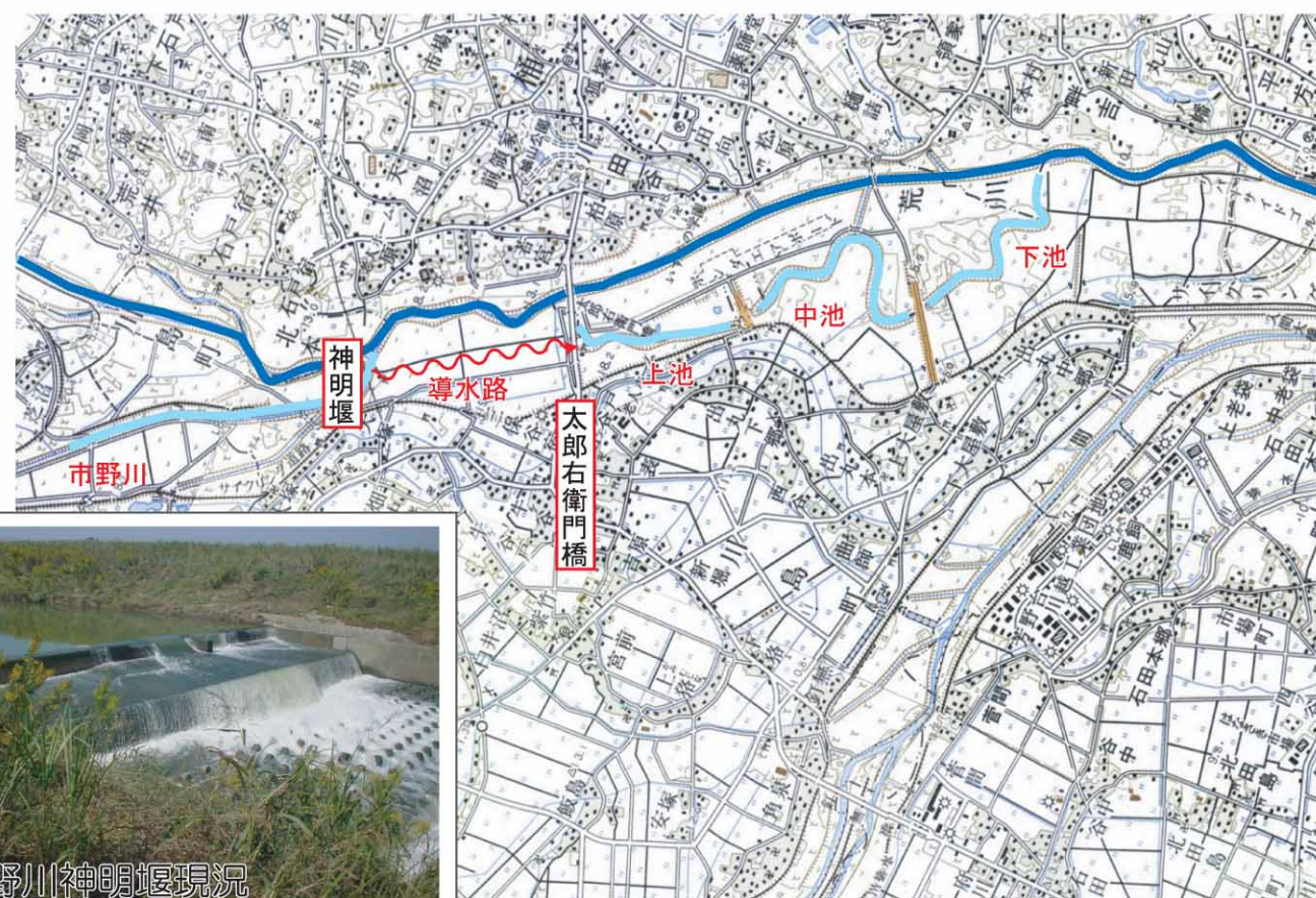
導水路平面図
