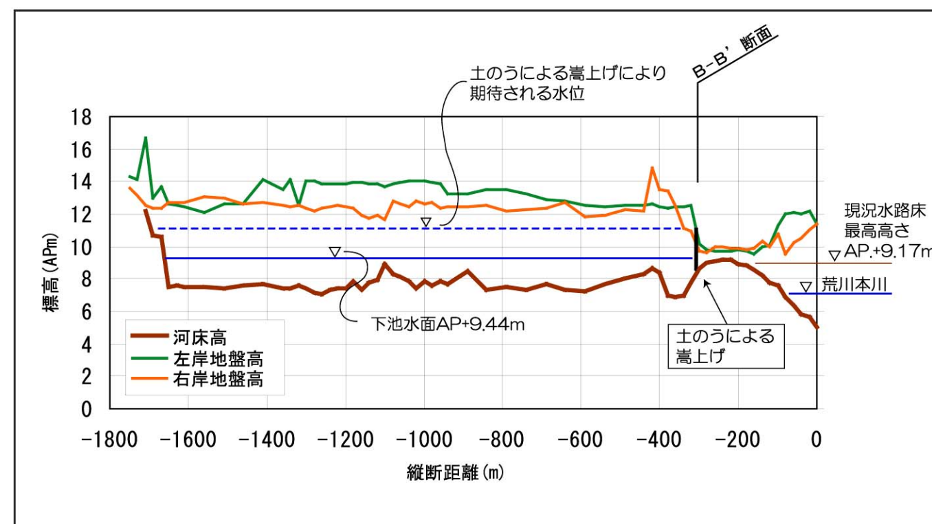
下池縦断面図
