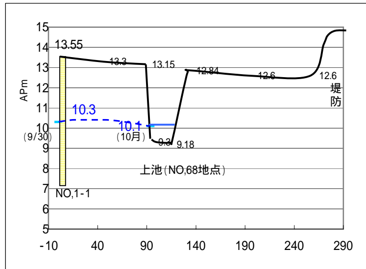
A-A'断面(上池横断)
