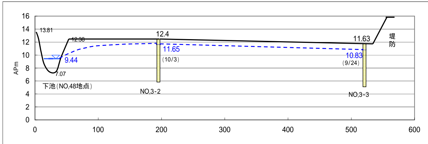
D-D'断面(下池~右岸堤防)
