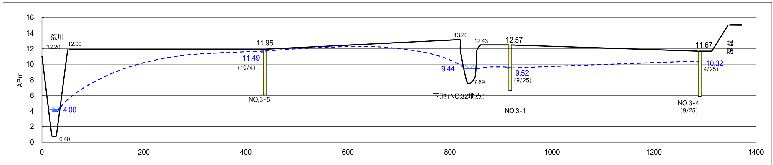
E-E'断面(荒川~下池~右岸堤防)
