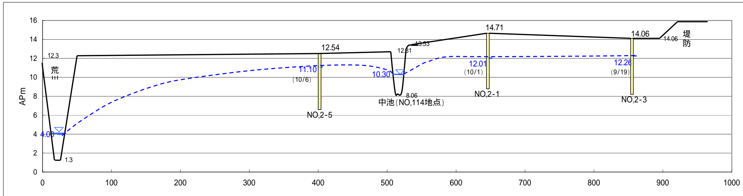
B-B'断面(荒川~中池~右岸堤防)
