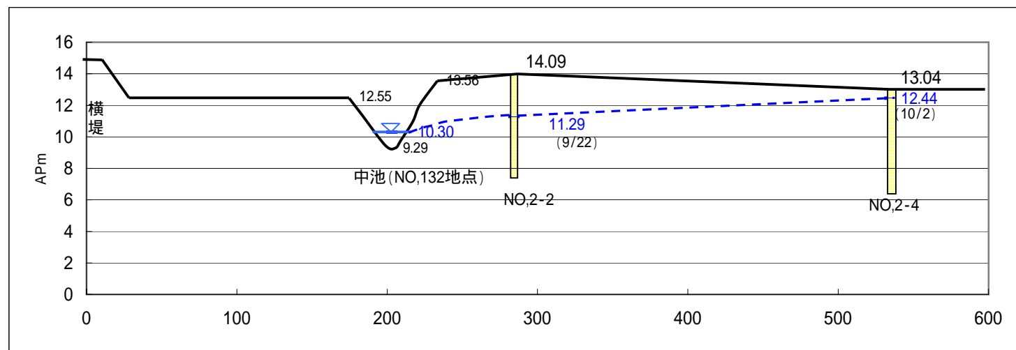
C-C'断面(横堤~中池)
