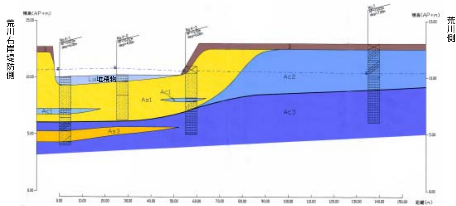
B - B' 断面（上池の横断図）
