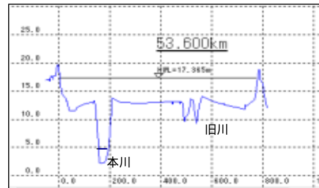
横断図
