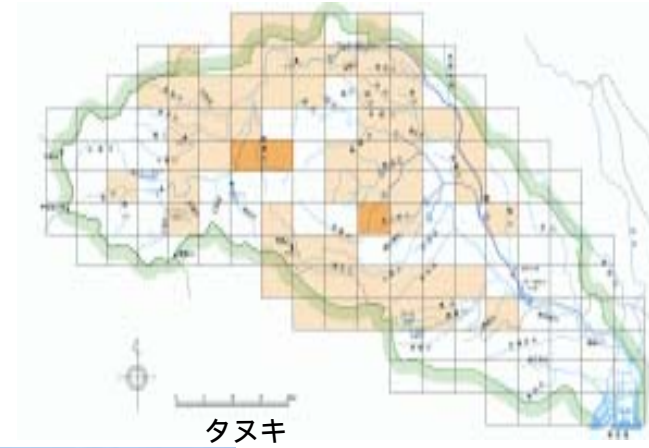
図-4 中型哺乳類の分布
