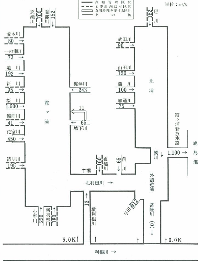
計画高水流量図
