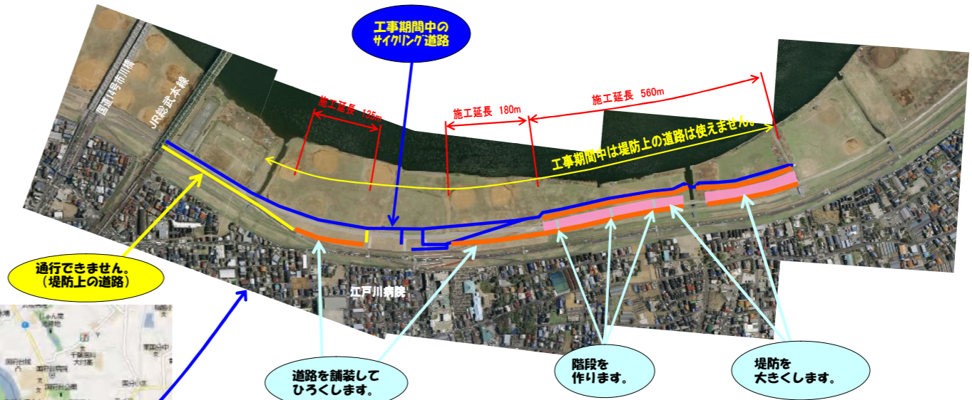
H19東小岩築堤工事全体図
