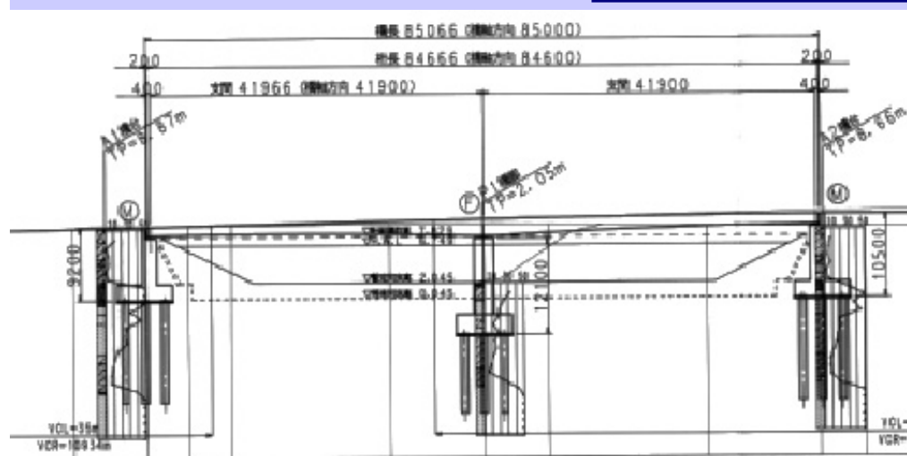
玉川橋一般図
