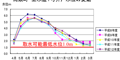
馬頭町 上水道1号井戸水位の変動
