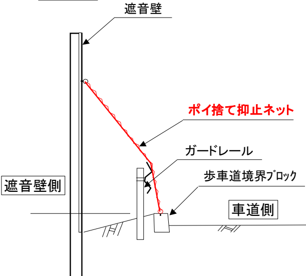
ゴミのポイ捨て抑止ネットの構造図
