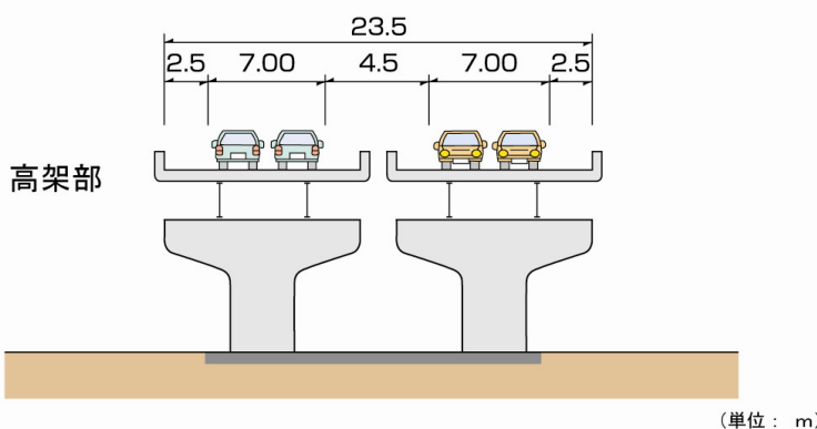
標準断面図
