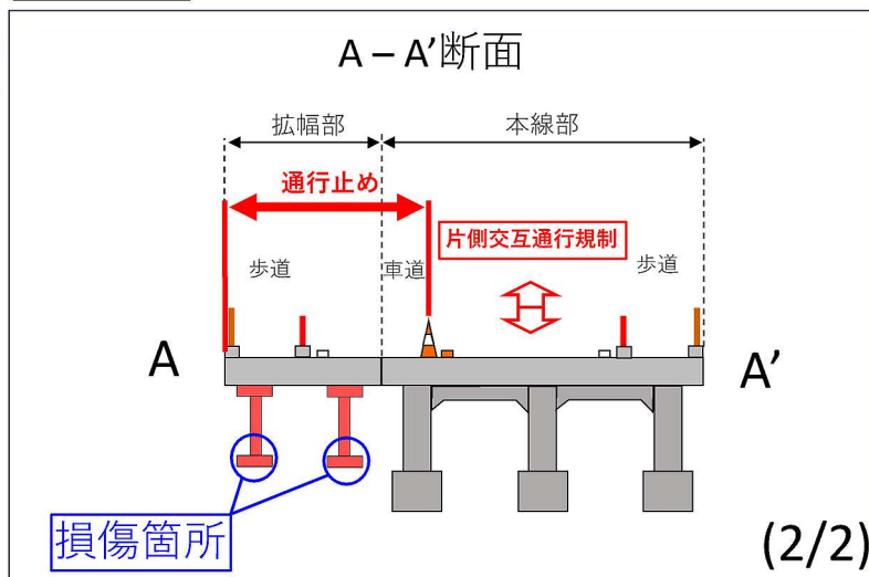
横断図
