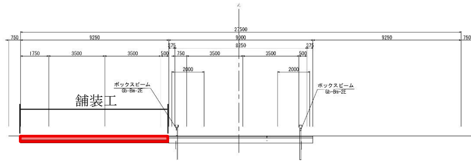
横断図 A-A'
