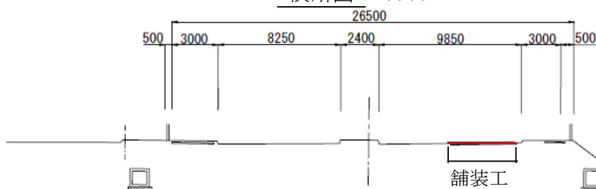
横断図 A-A'
