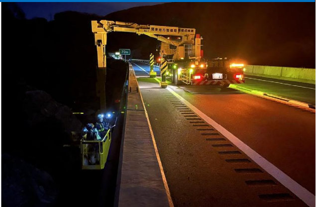
橋梁点検車による点検のイメージ写真 中部横断自動車道の点検時の写真です。
