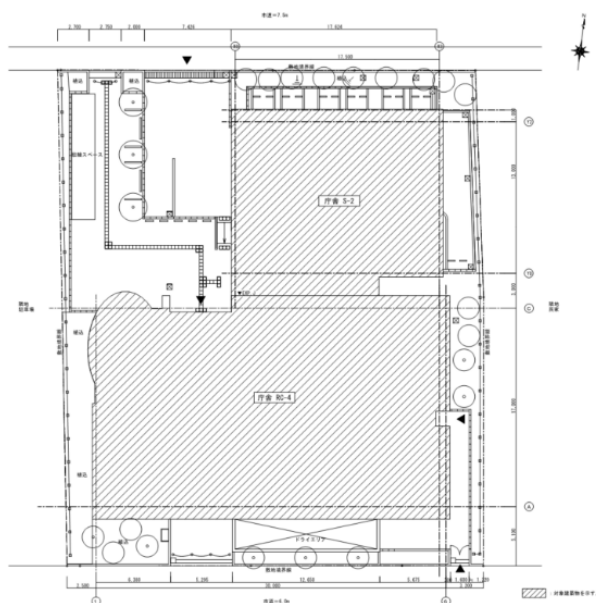
配置図
