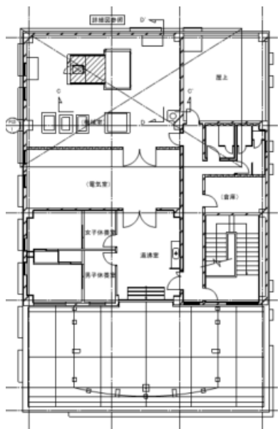
3階平面図（改修前）
