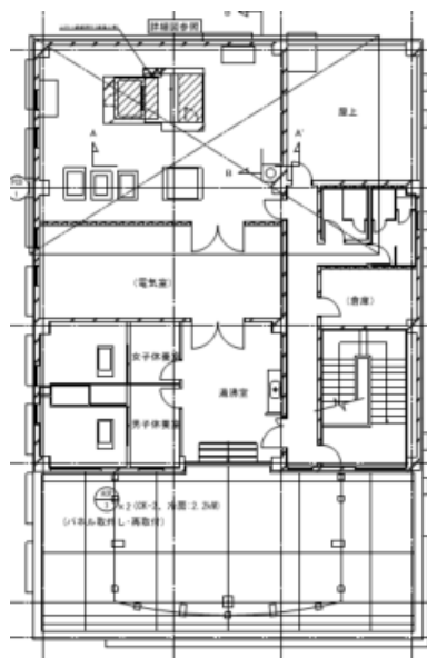
3階平面図（改修後）
