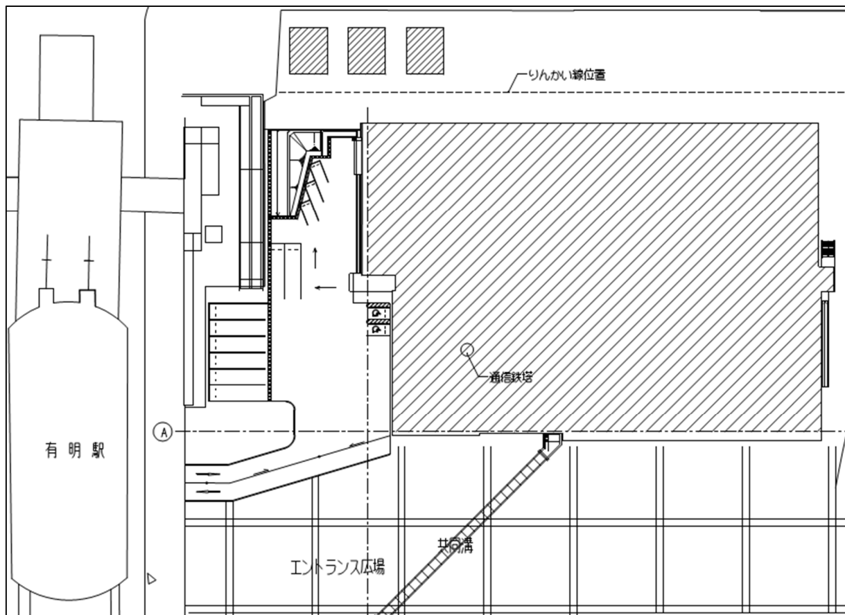
配置図
