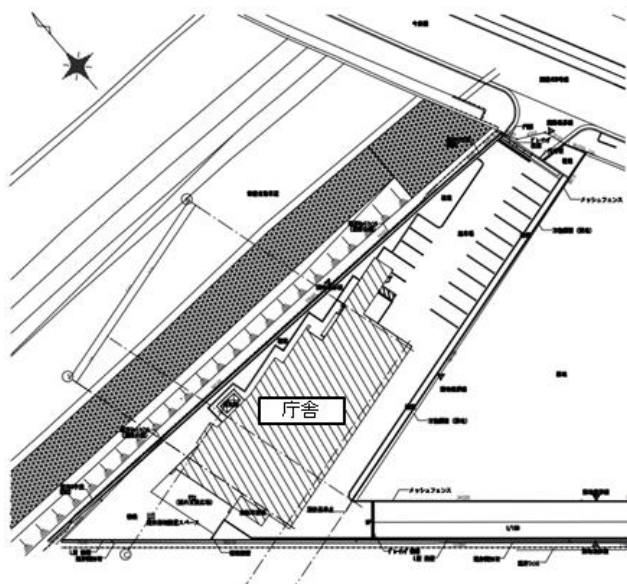
配置図
