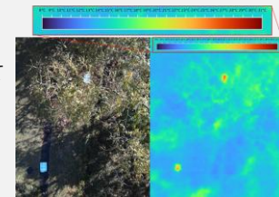
図-1 熱源の抽出に関する検討
