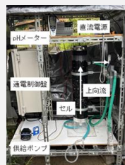
図1 中和処理装置
